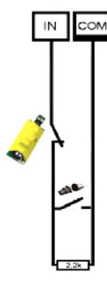
шлейф с оконечным резистором
